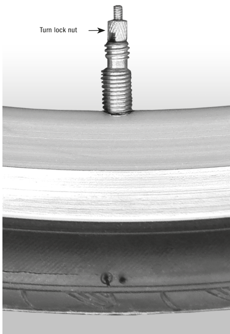
Fig. 14 - Presta valve
